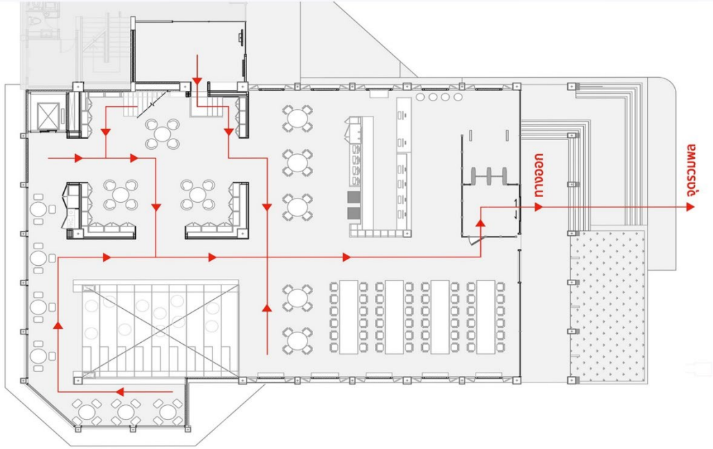
แผนผังเส้นทางหนีไฟอาคารหอสมุดวังท่าพระ (ชั้น 1)
